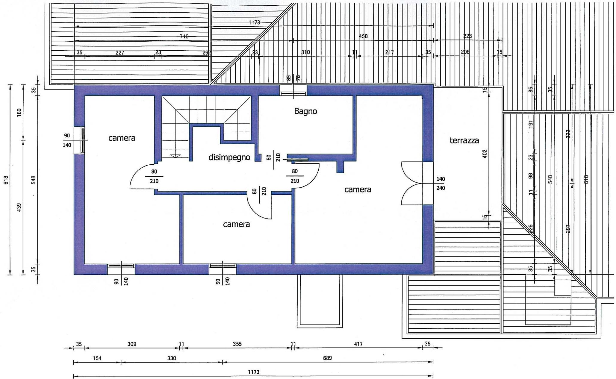
Pianta Piano Secondo - Scala 1 : 50
